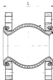
COMPENSATEUR DE DILATATION EXPANSION JOINT
