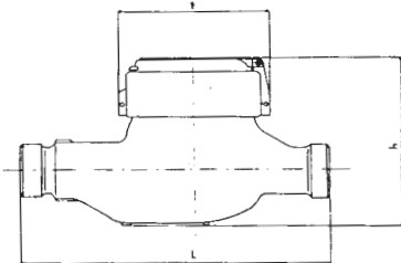
COMPTEURS JETS MULTIPLES MULTI-JET WATER METER
