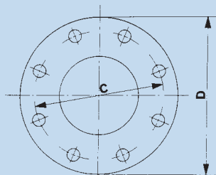
BRIDES EN ACIER STEEL FLANGES
