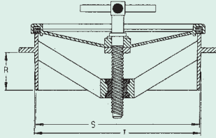
VANNE CLAPET TILTING WEIR GATE
