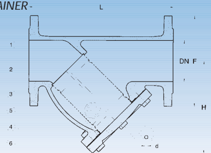
FILTRE BB STRAINER -
