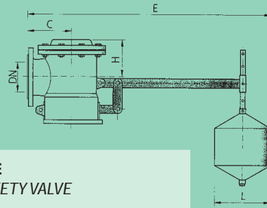
ROBINET FLOTTEUR FLOAT VALVE
