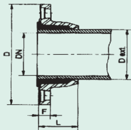
RACCORDS EN LAITON A SERRAGE EXTERIEUR BRASS FITTINGS FOR UPVC PIPES
