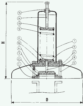
OBTURATEUR A FLOTTEUR EQUILIBRATED FLOAT VALVE
