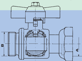
ROBINET AVANT OU APRES COMPTEUR METER COCK
