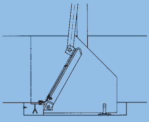
VANNE CLAPET TILTING WEIR GATE
