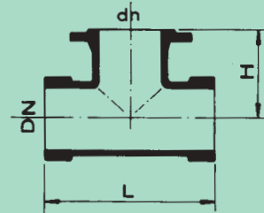
RACCORDS EN FONTE POUR AMIANTE CIMENT CAST IRON FITTINGS FOR AC PIPES
