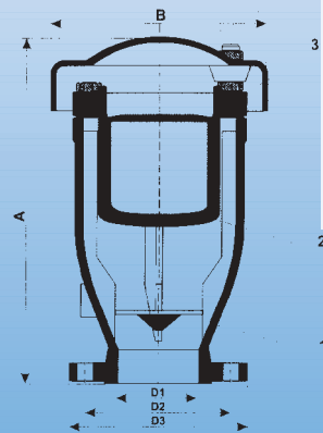
VENTOUSE 2 FONCTIONS DOUBLE ACTION AIR RELEASE VALVE
