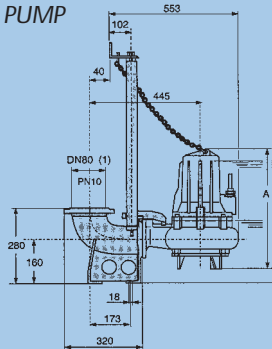
GRUPE MOTOPOMPE MOTOR PUMP SET
