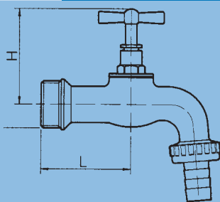
ROBINET DE PUISAGE SPHERIQUE BALL BIBCOCK HOSE COUPLING
