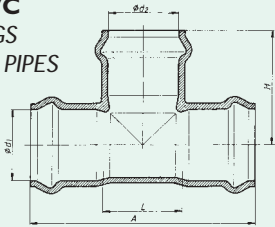
RACCORDS EN FONTE POUR TUBE FONTE DI FITTINGS FOR DI PIPES
