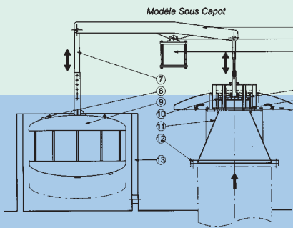
OBTURATEUR A FLOTTEUR EQUILIBRATED FLOAT VALVE
