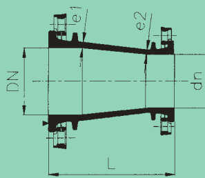
RACCORDS EN FONTE A BRIDES DI FLANGED FITTINGS
